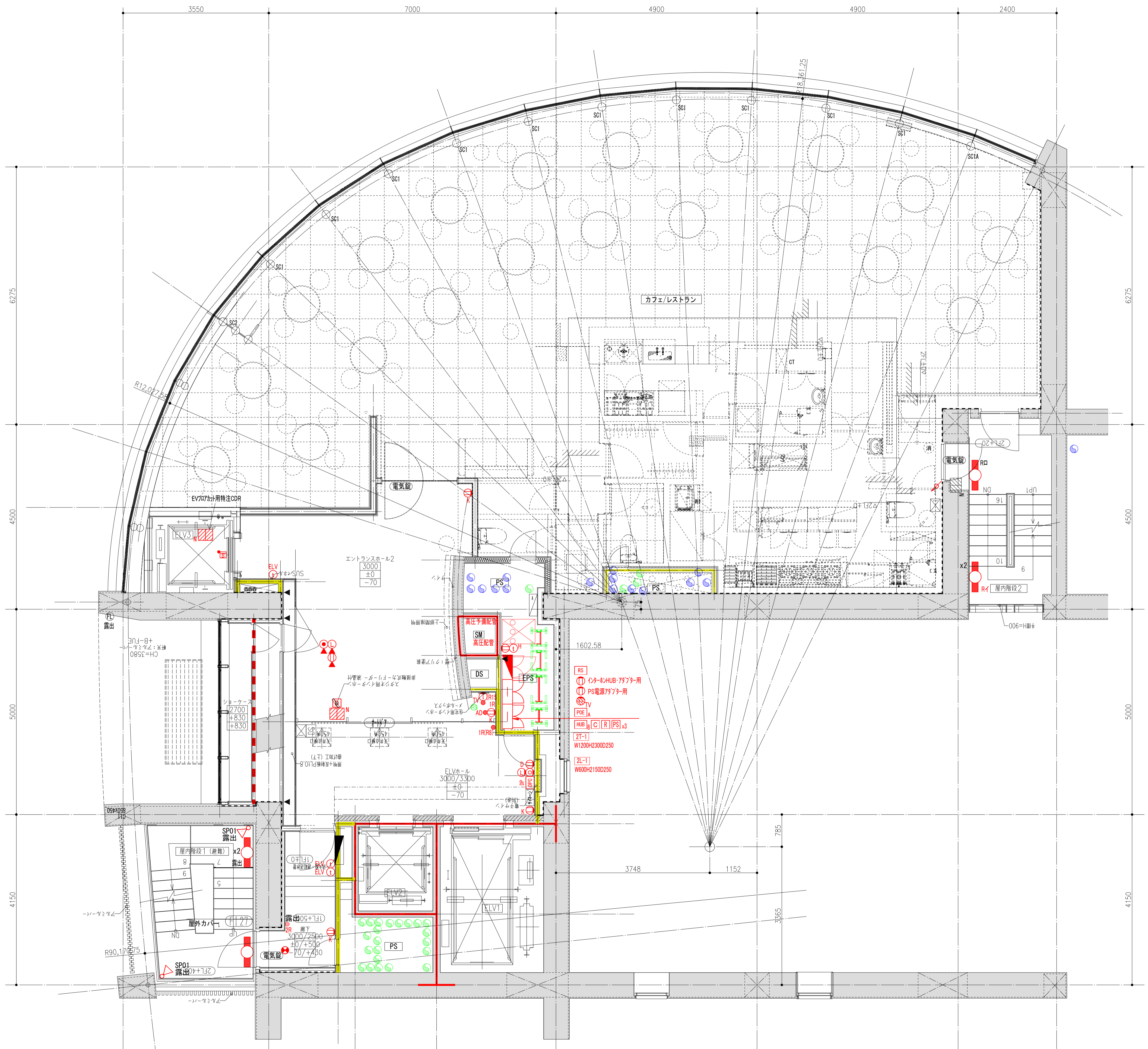
商業ビル 飲食店 床・壁総合図 1:50(A1)
