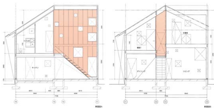
断面図
