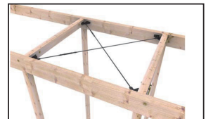
水平ブレースの例 タナカ住宅資材カタログより
